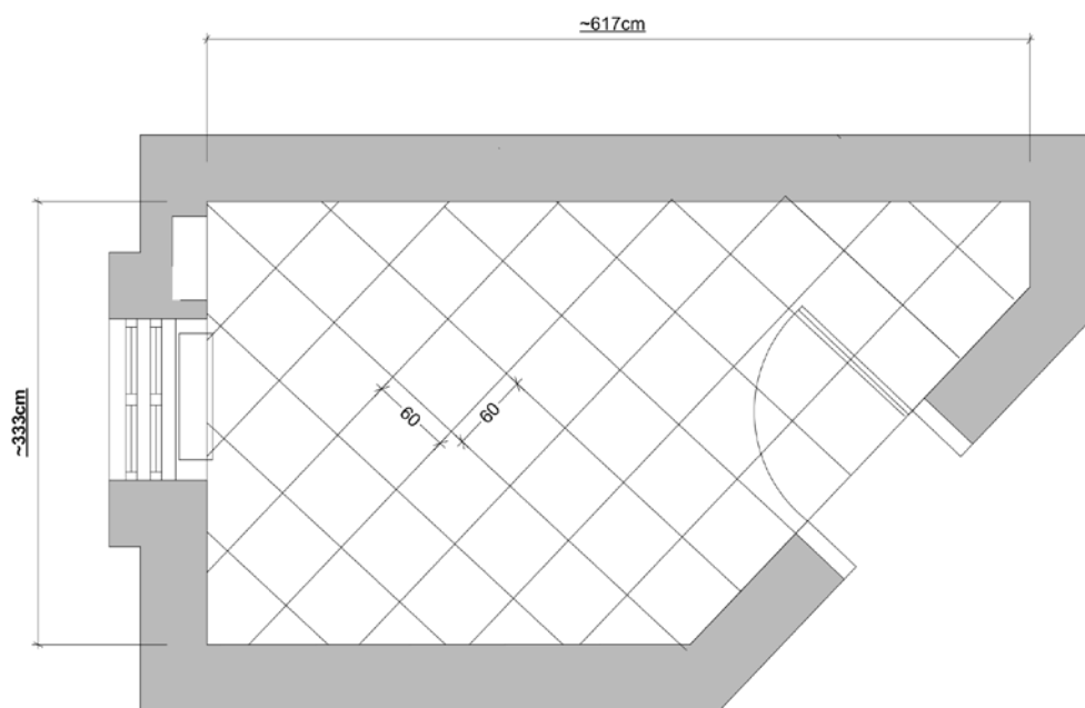
Osnova granitne keramike r=1:50
