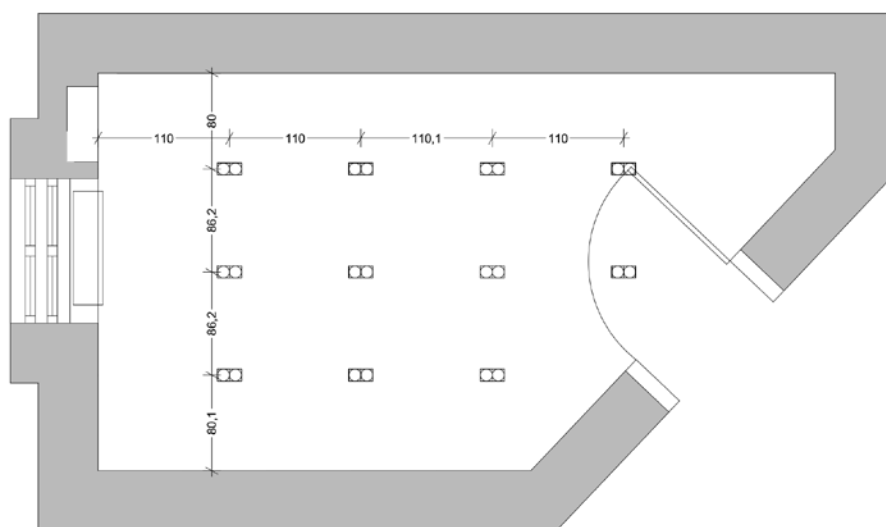
Osnova spuštenog plafona sa osvetljenjem R=1:50
